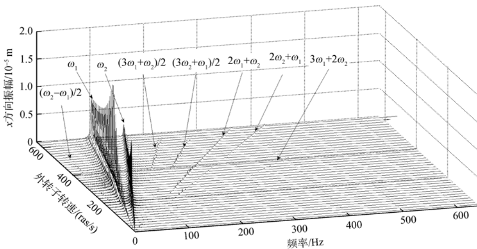
图 7 盘 3 的三维频谱图(游隙为 6\mu\text{m} ) Fig. 7 3-D spectrogram of disk 3 (clearance of 6\mu\text{m} )
