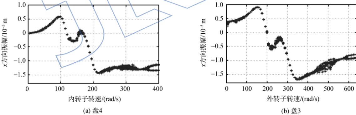
图12 盘4和盘3随转子转速分岔图(径向游隙为 10\mu\text{m} )
