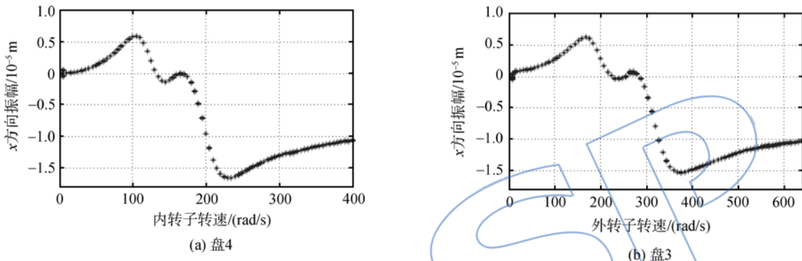
图11 盘4和盘3随转子转速分岔图(径向游隙为 2\mu\text{m} )
