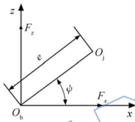
图2 挤压油膜阻尼器轴颈中心与油膜环中心的相对关系
